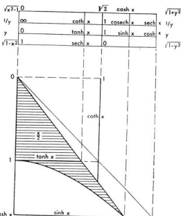
Hyperbelfunktionen Die Skalen dieses Bildes sind nicht logarithmiert
