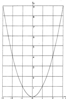
Quadratische Einheitsparabel y = x^2
